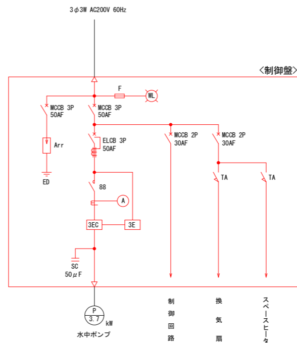
単線結線図
