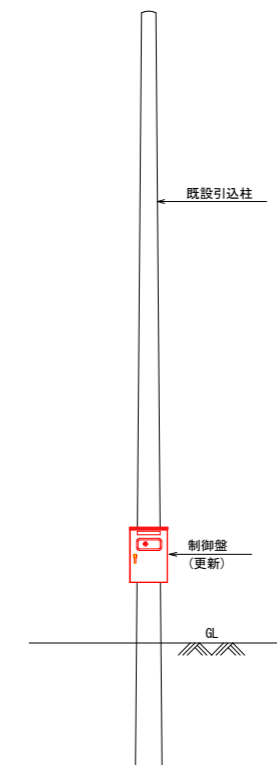
制御盤据付参考図 S=1/50
